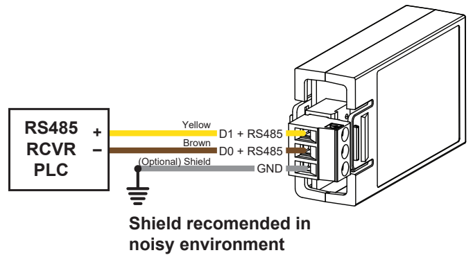
Modbus Module
